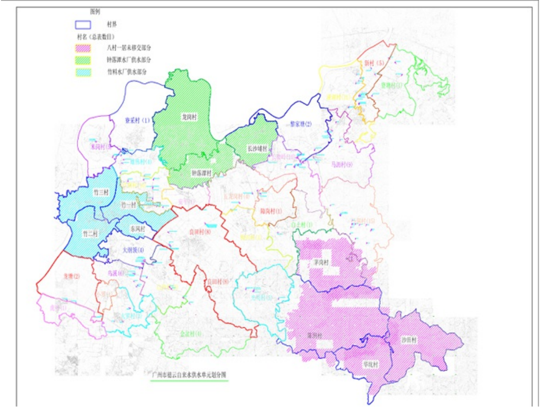
供水区域示意图
