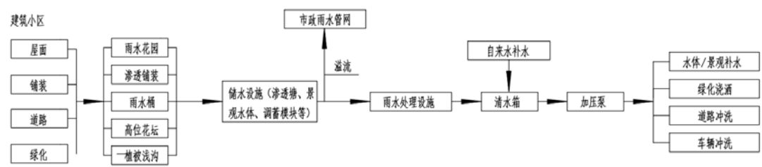
图 J-14 雨水收集利用典型工艺流程图
