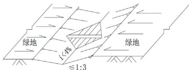
图 J-7 转输型三角形断面植草沟典型构造示意图
