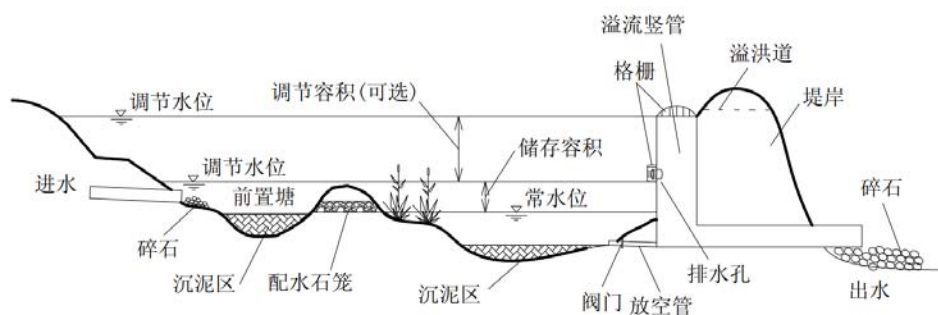
图 J-9 湿塘典型构造示意图
