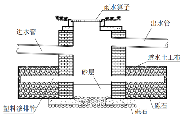
图 J-6 辐射渗井构造示意图
